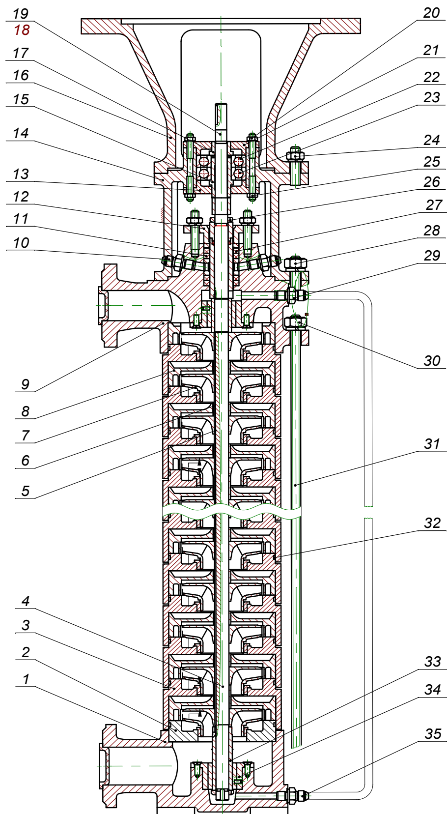
Рисунок 1 Разрез насоса
